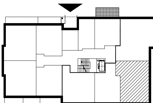
SCHEMAT KONDYGNACJI 1:500
